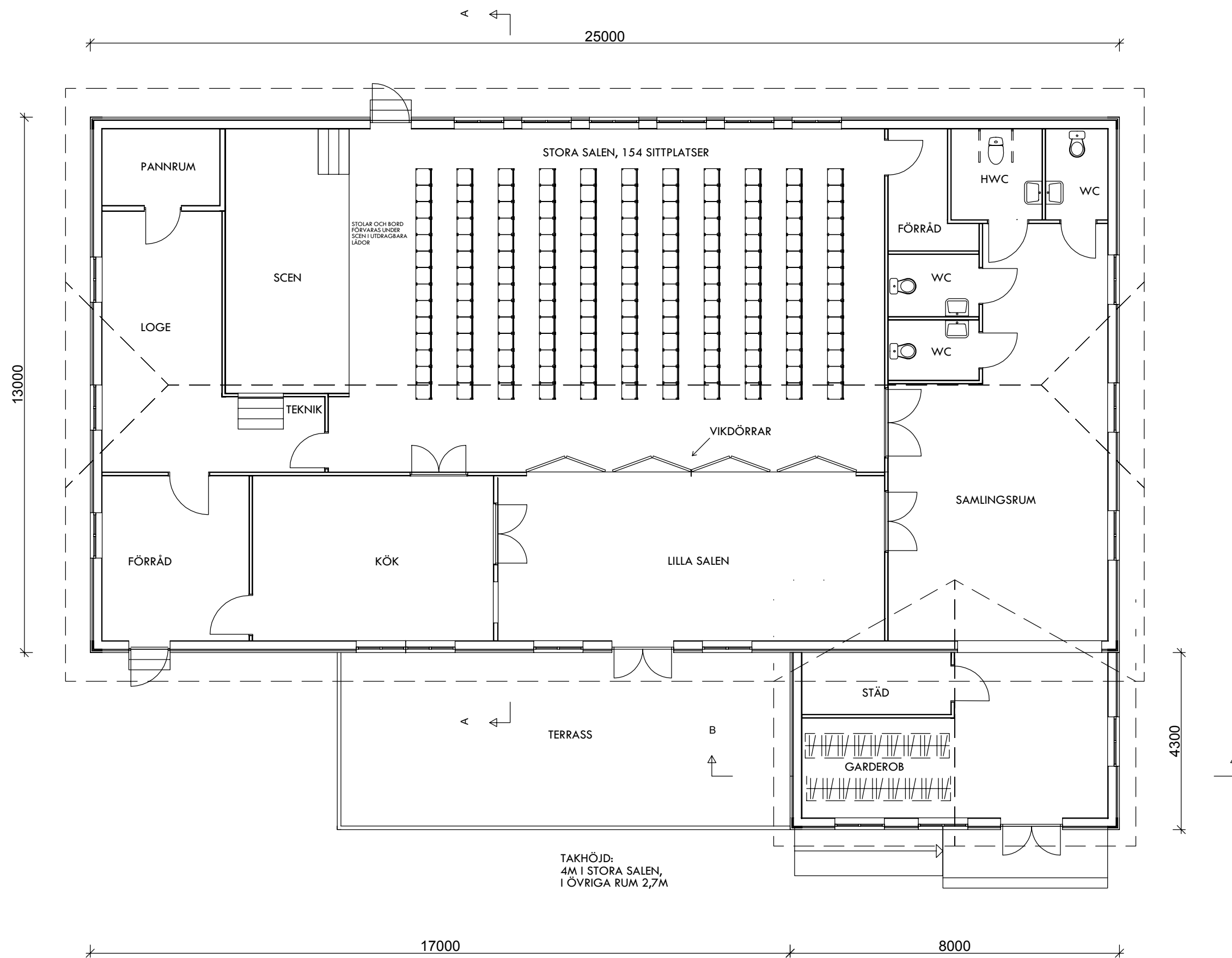
PLAN SKALA 1:100
